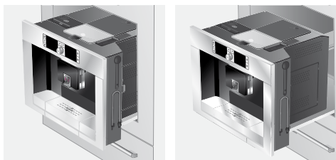
Auszugsposition 1 Auszugsposition 2
